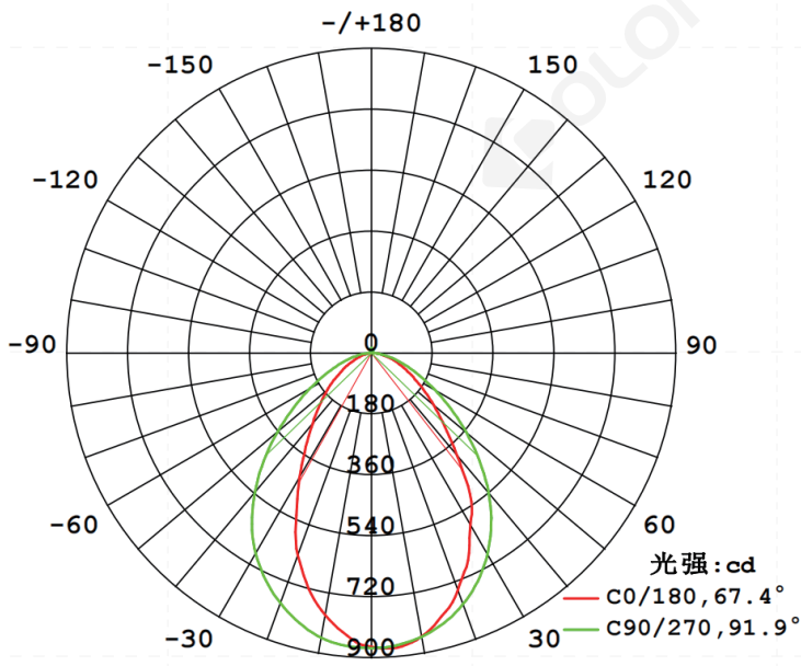
配光曲线图
